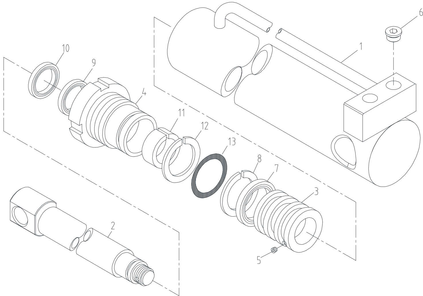
익스펜딩 실린더 조립체 Fig. 4-2 SCS886 EXPANDING CYL' ASS'Y
