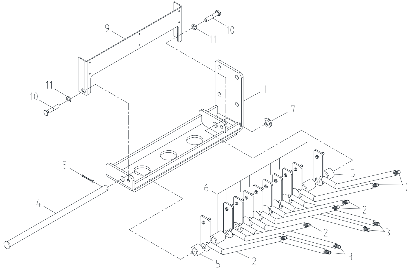
레버 스텐드 세트 Fig. 3-2-2 SCS886 LEVER STAND SET
