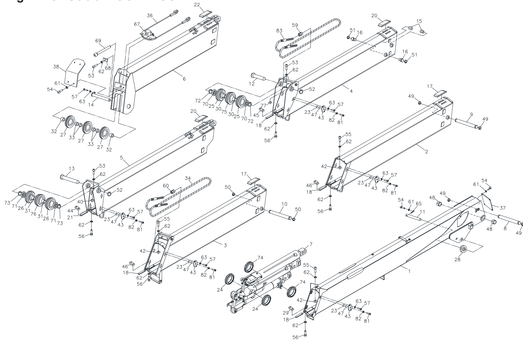
붐 조립체 Fig. 1 SCS886 BOOM ASS'Y
