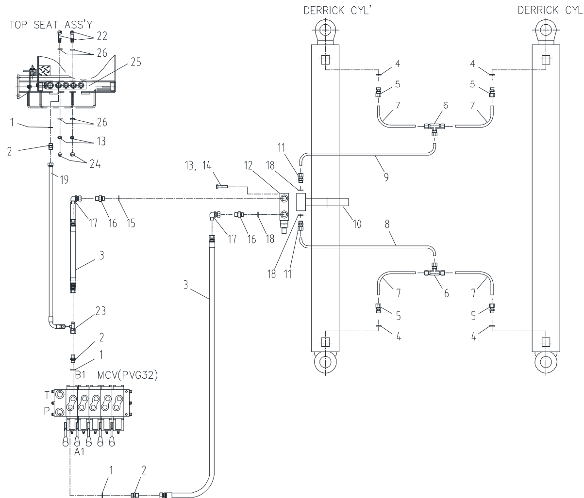
데릭 배관 Fig. 5-2 SCS886 DERRICK PIPING
