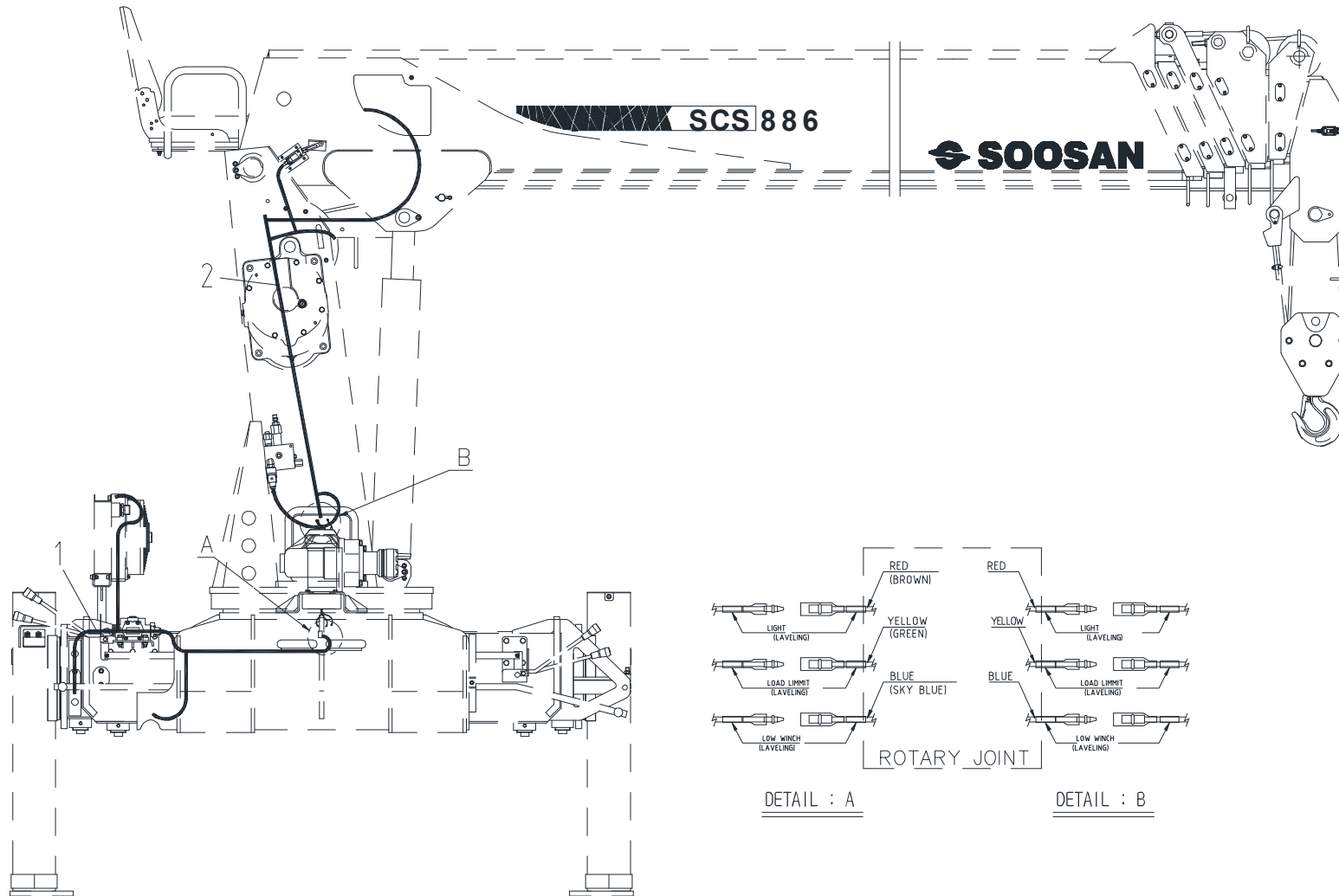
전선 조립체 Fig. 10 SCS886 WIRING ASS'Y
