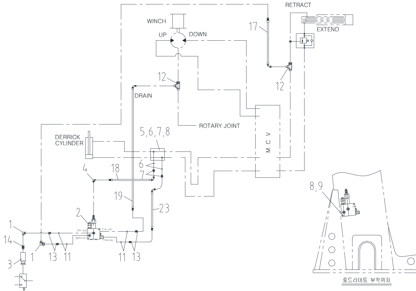
과하중방지 배관 조립체 Fig. 5-7 SCS886 OVERWINDING ALARM PIPING ASS'Y
