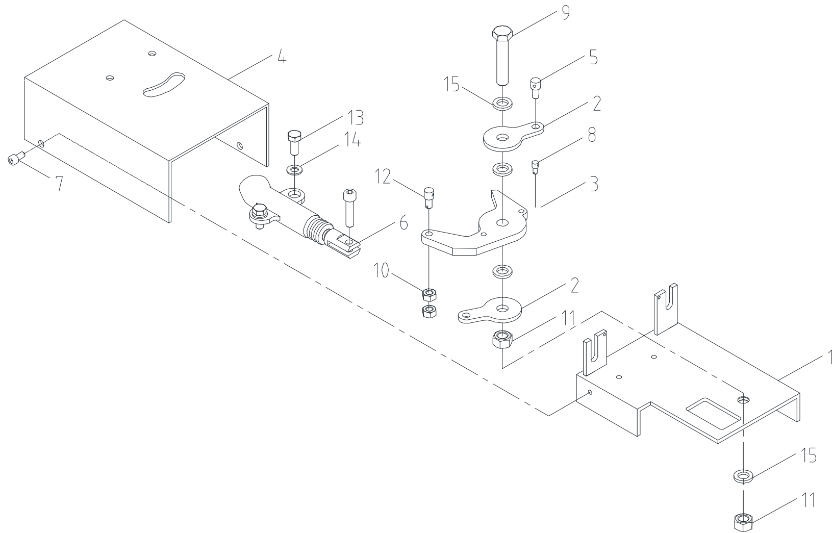
악셀 시스템 파트 Fig. 9-3 SCS886 ACC'L SYSTEM PART
