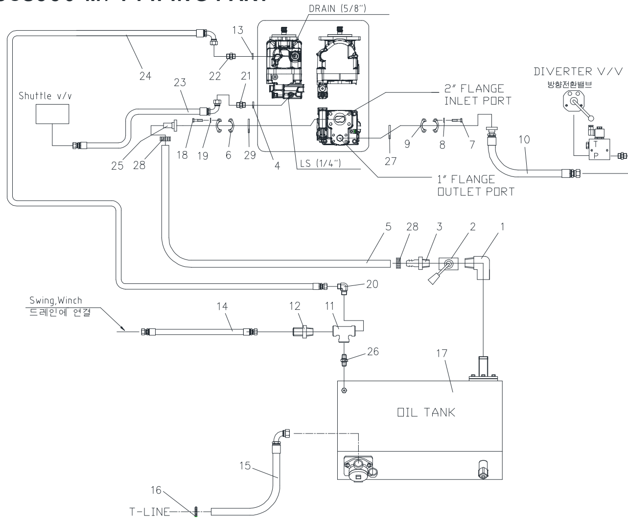
장착 배관 파트 Fig. 9-6 SCS886 M / T PIPING PART
