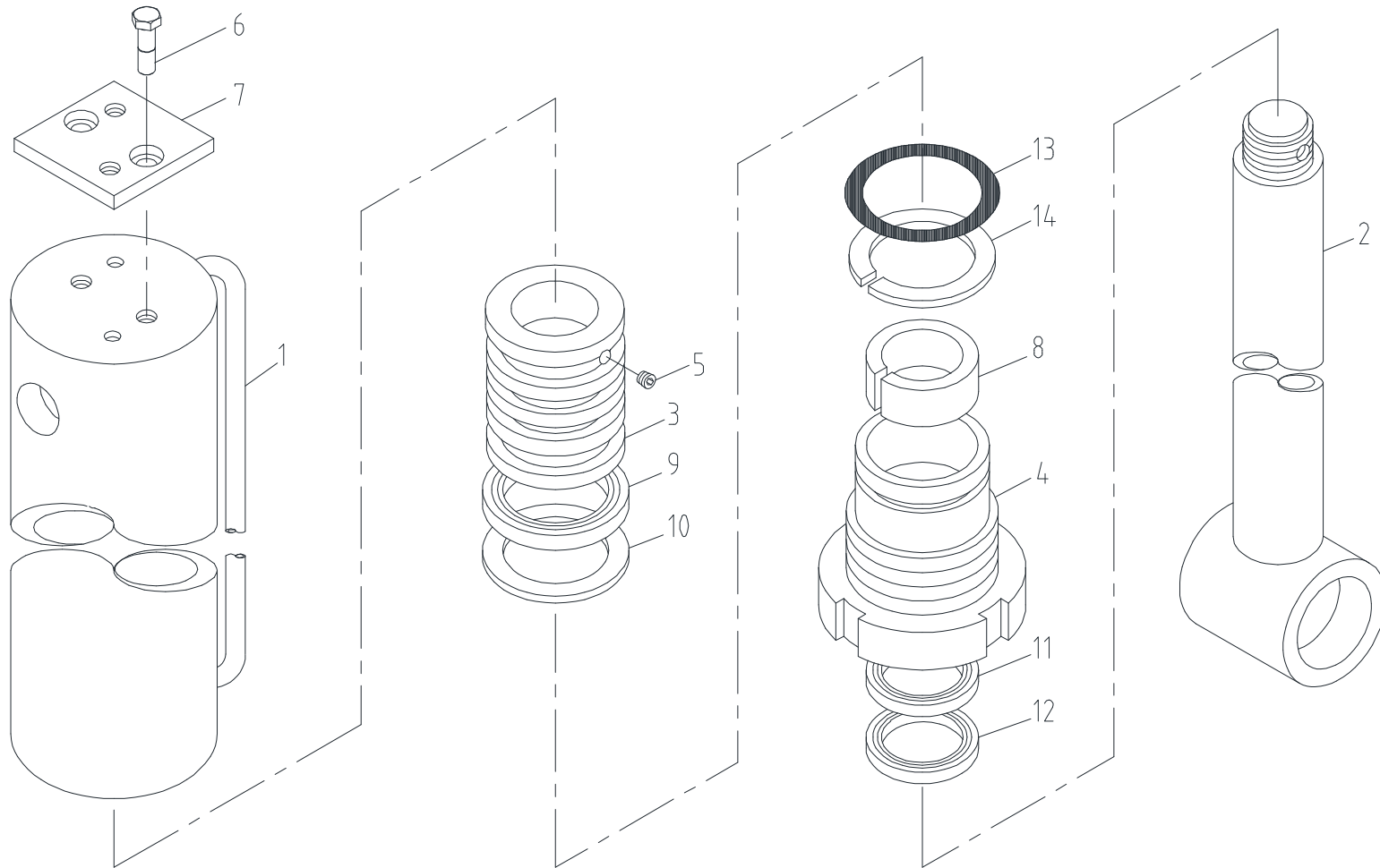
잭 실린더 조립체 Fig. 4-1 SCS886 JACK CYL' ASS'Y
