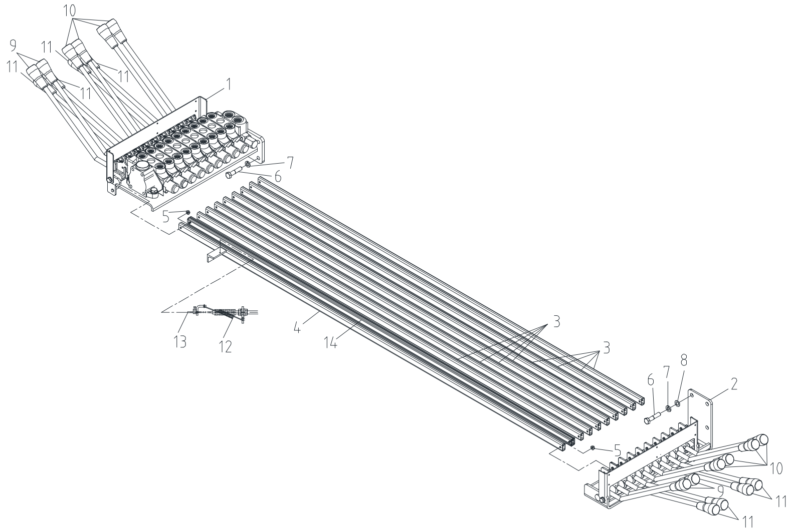
오퍼레이션 조립체 Fig. 3-2 SCS886 OPERATION ASS'Y
