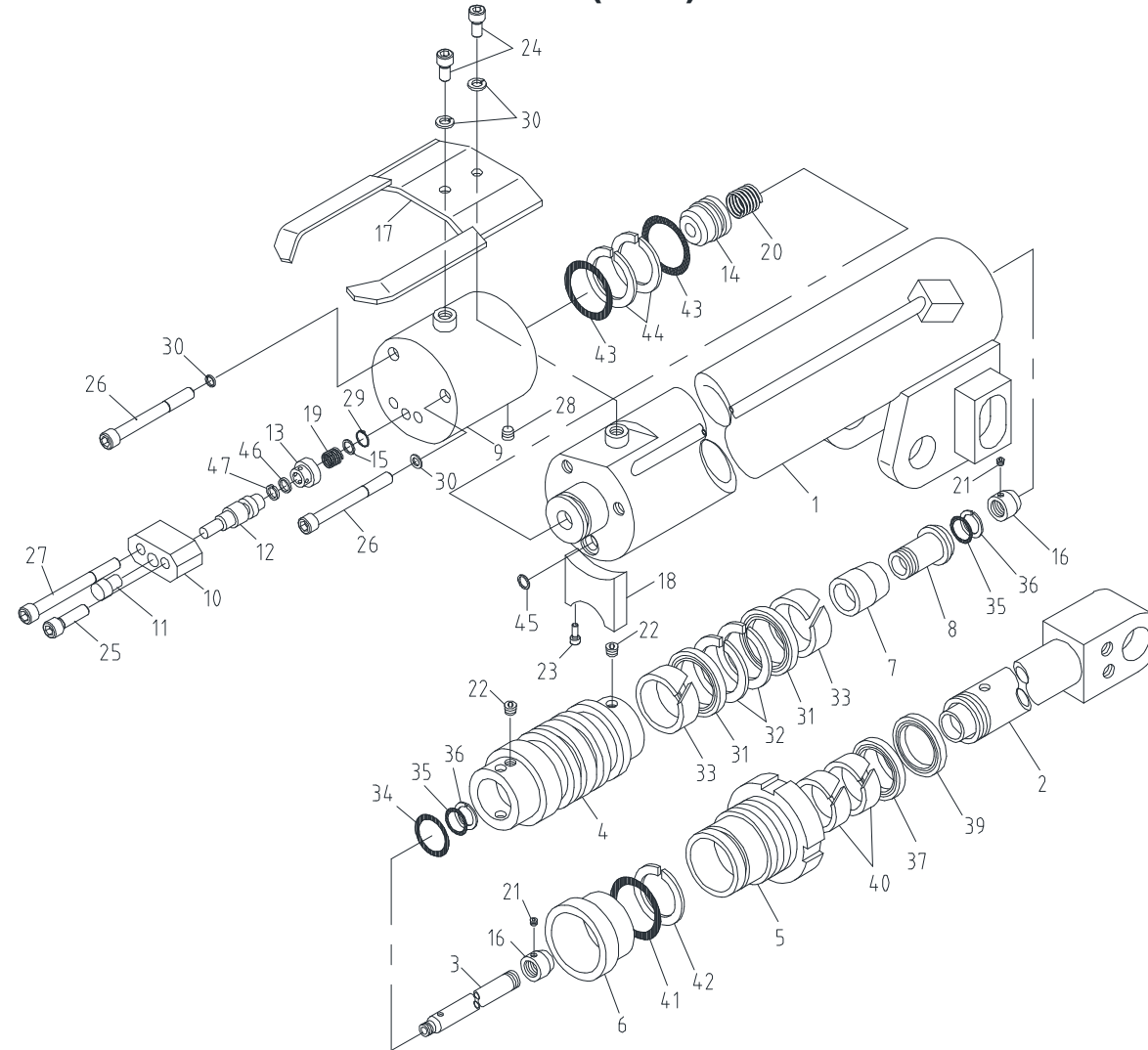
텔레스코픽 실린더(1 단) 조립체 Fig. 1-1-1 SCS887 TELESCOPIC CYL'(1st) ASS'Y
