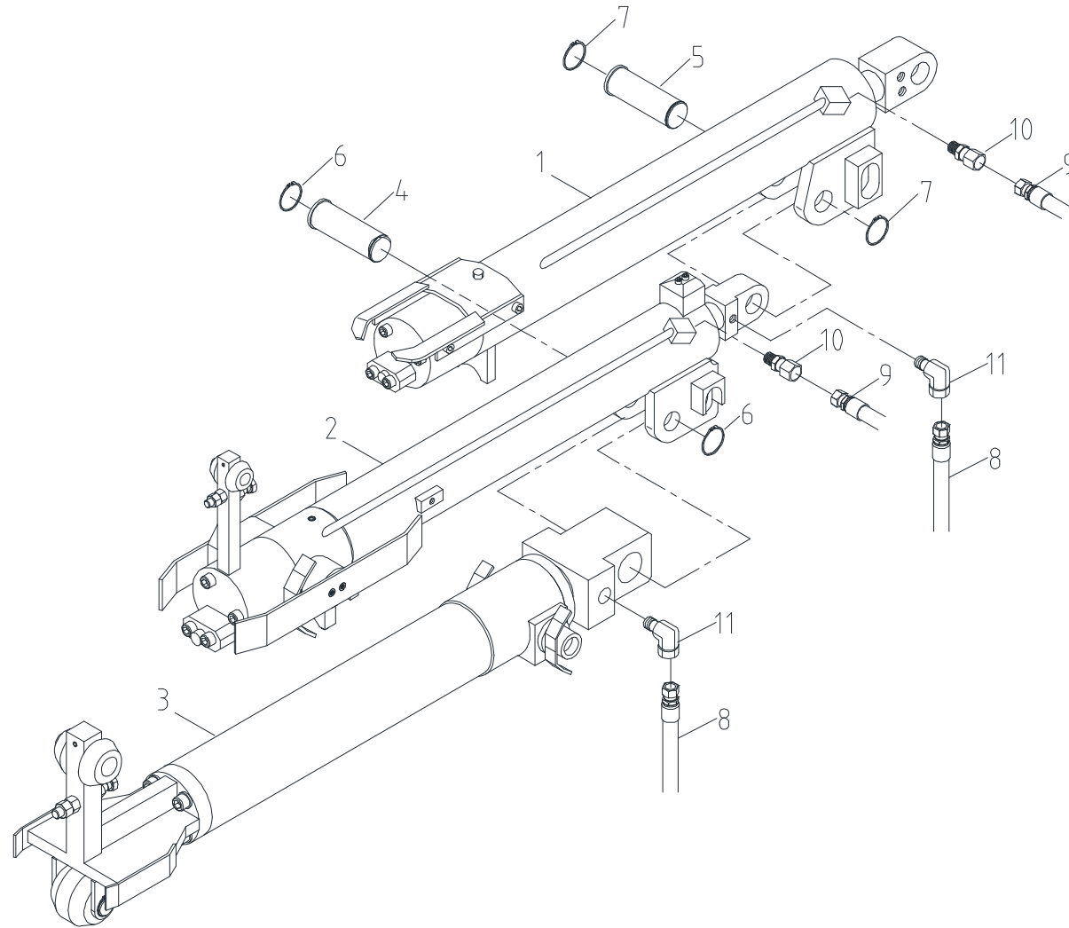
텔레스코픽 실린더 조립체 Fig. 1-1 SCS887 TELESCOPIC CYL' ASS'Y
