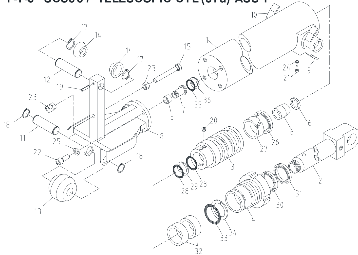
텔레스코픽 실린더(3단) 조립체 Fig. 1-1-3 SCS887 TELESCOPIC CYL'(3rd) ASS'Y
