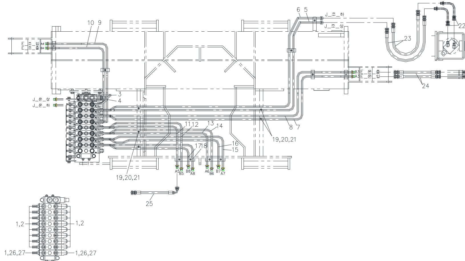
아우트리거 배관 Fig. 5-6 SCS886 OUTRIGGER PIPING
