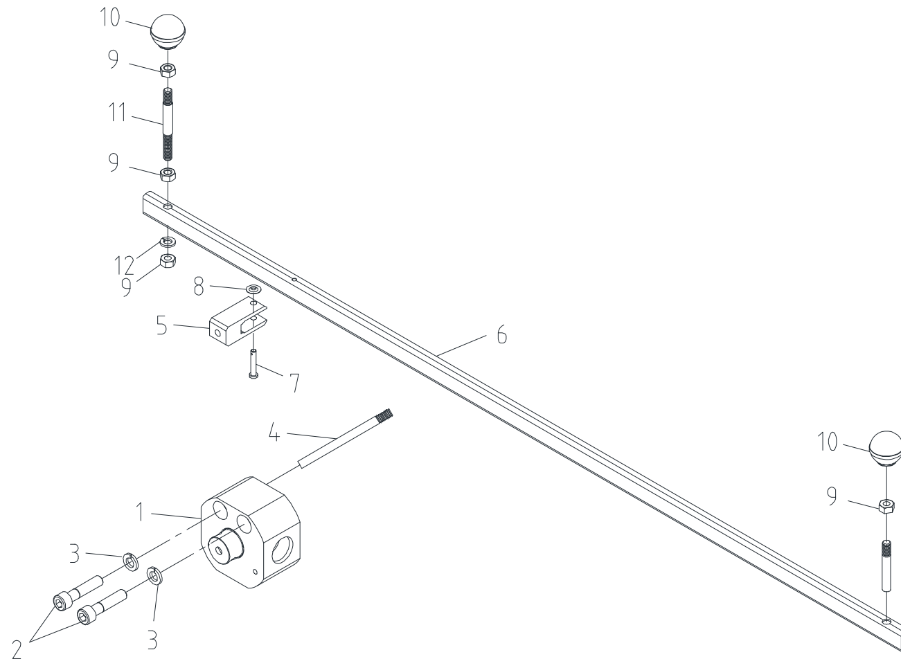
디버터 밸브 세트 Fig. 3-3 SCS886 DIVERTER V/ V SET
