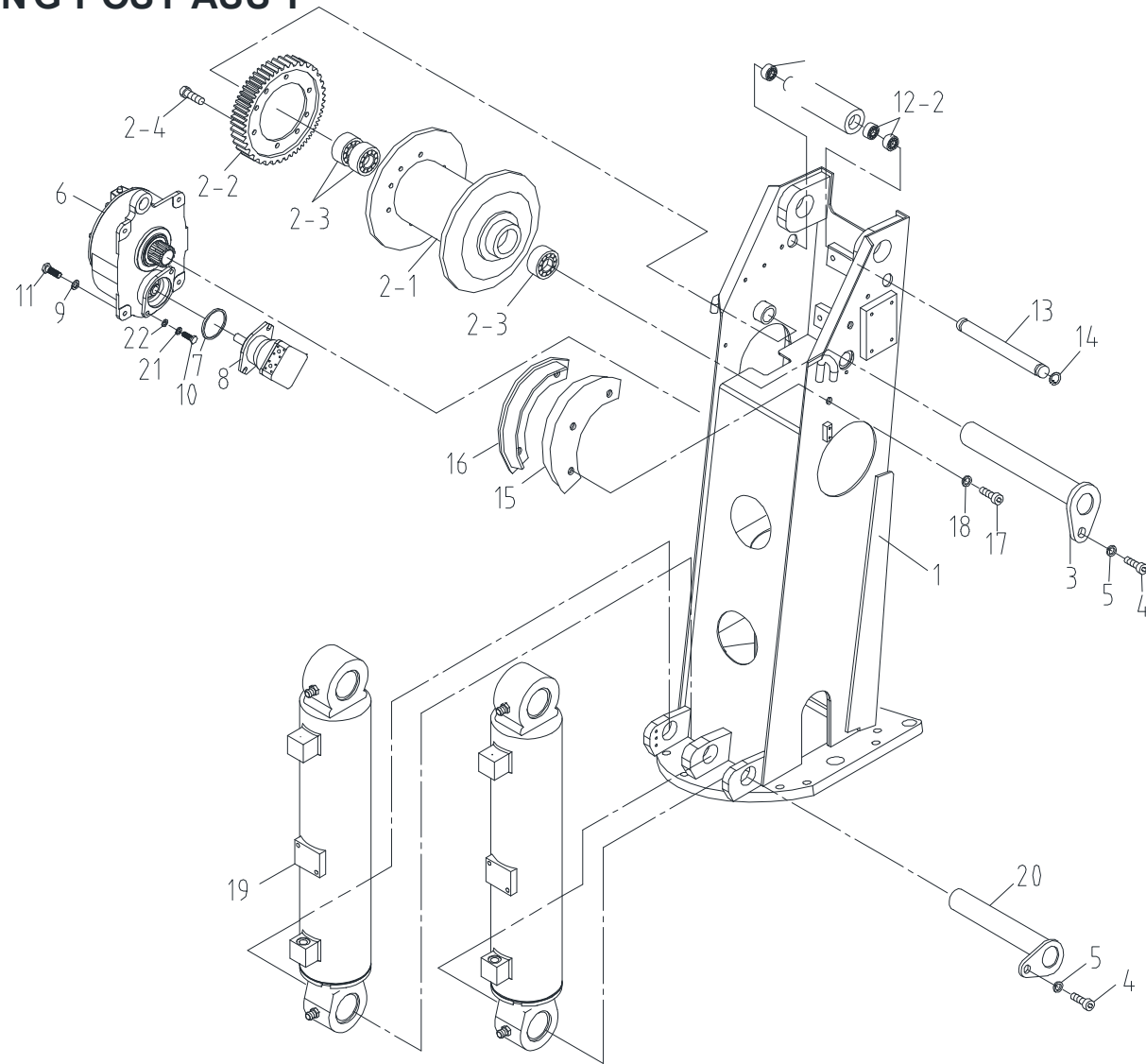
스윙 포스트 조립체 Fig. 2 SCS886 SWING POST ASS'Y
