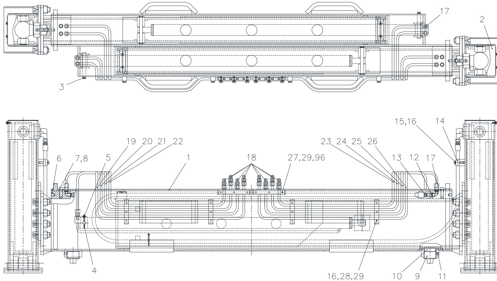
후방 아웃트리거 조립체 Fig. 9-2-1 SCS886 REAR OUTRIGGER ASS'Y
