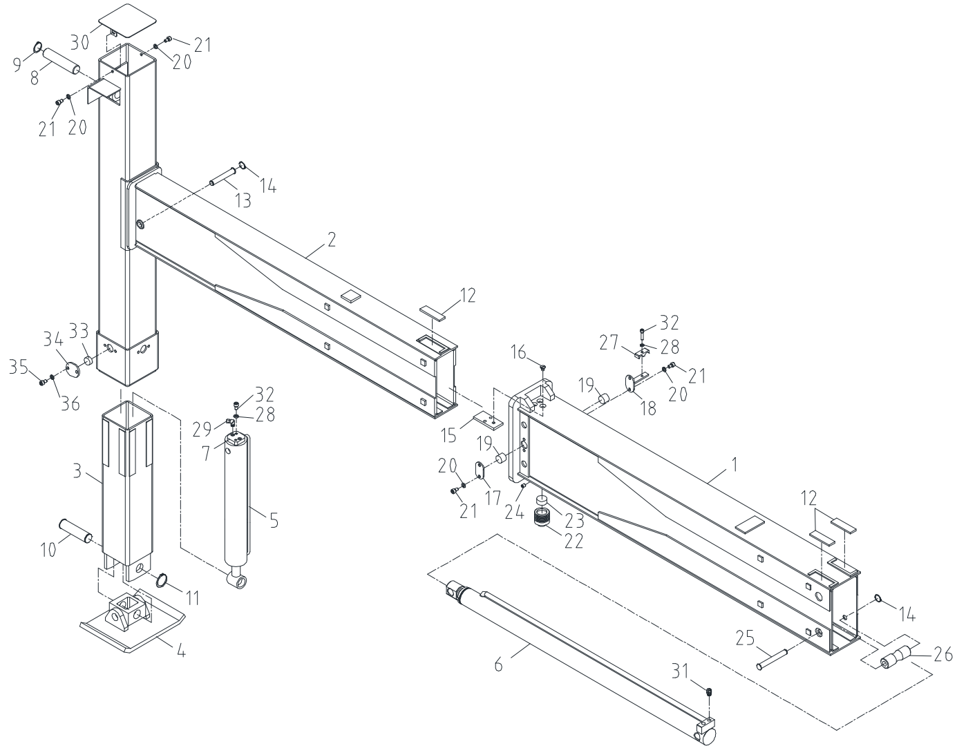
아우트리거 조립체 Fig. 4 SCS886 OUTRIGGER ASS'Y
