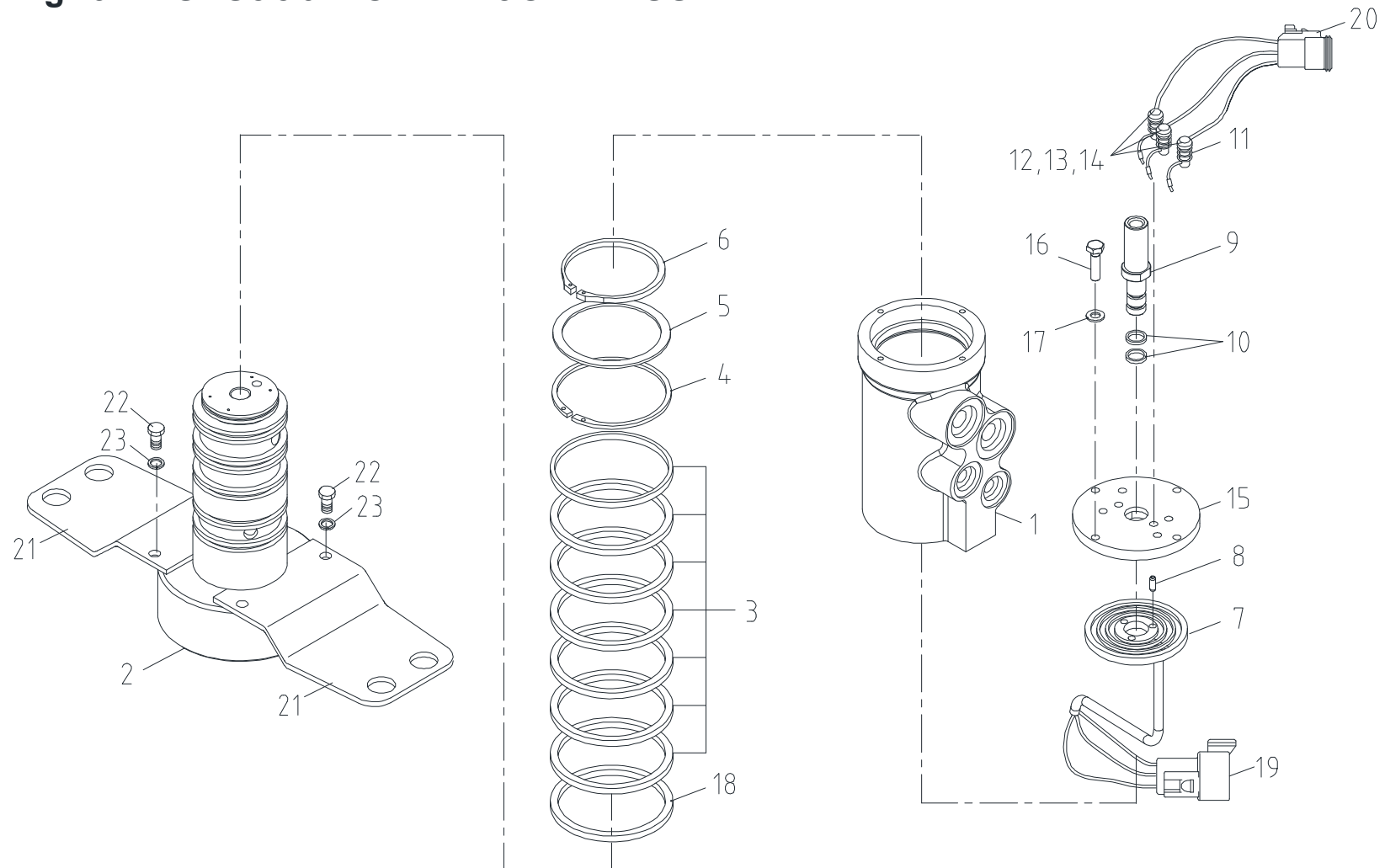
로타리 조인트 조립체 Fig. 3-1 SCS886 ROTARY JOINT ASS'Y
