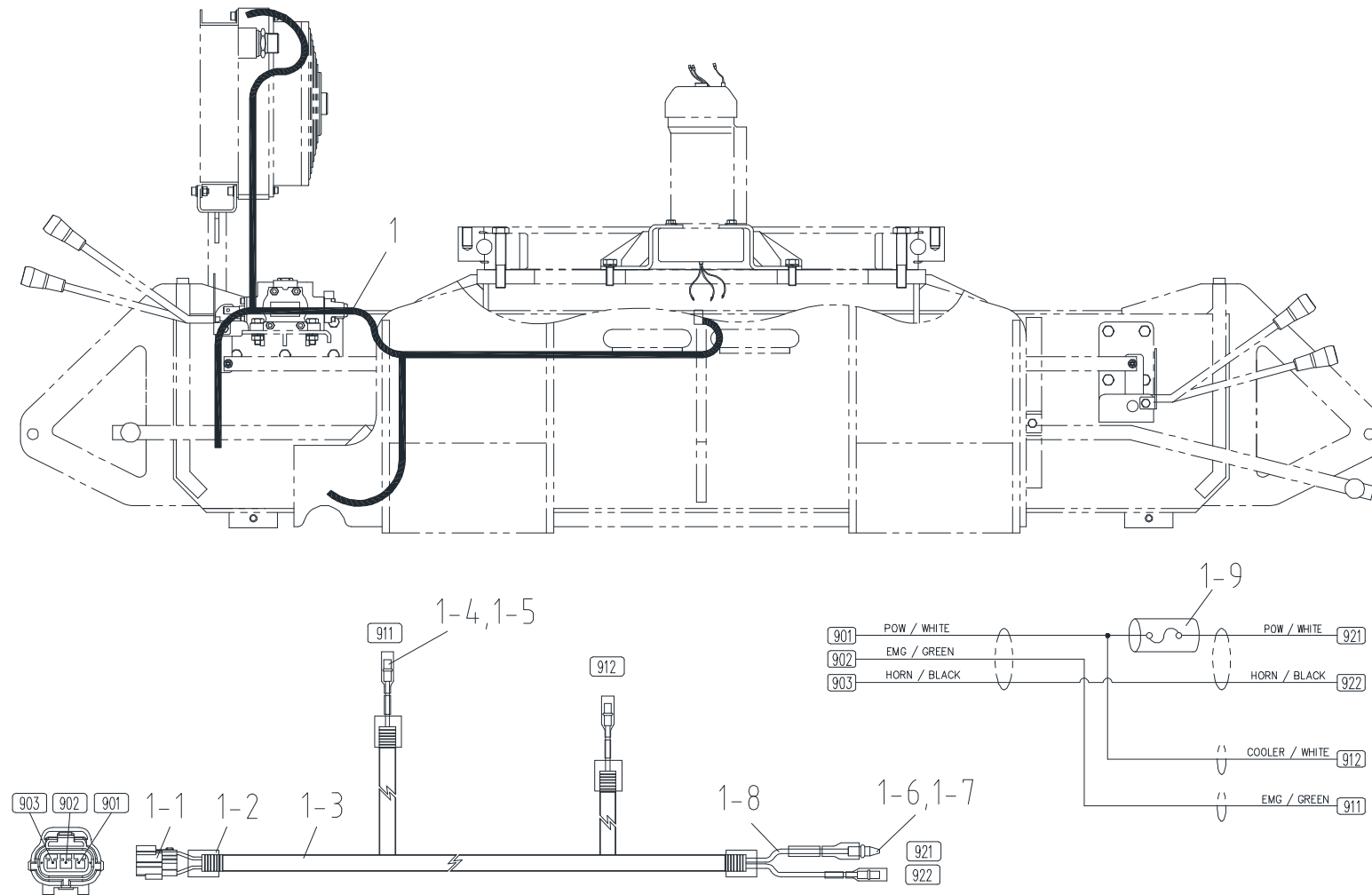
프레임 전선 Fig. 10-1 SCS886 FRAME WIRING
