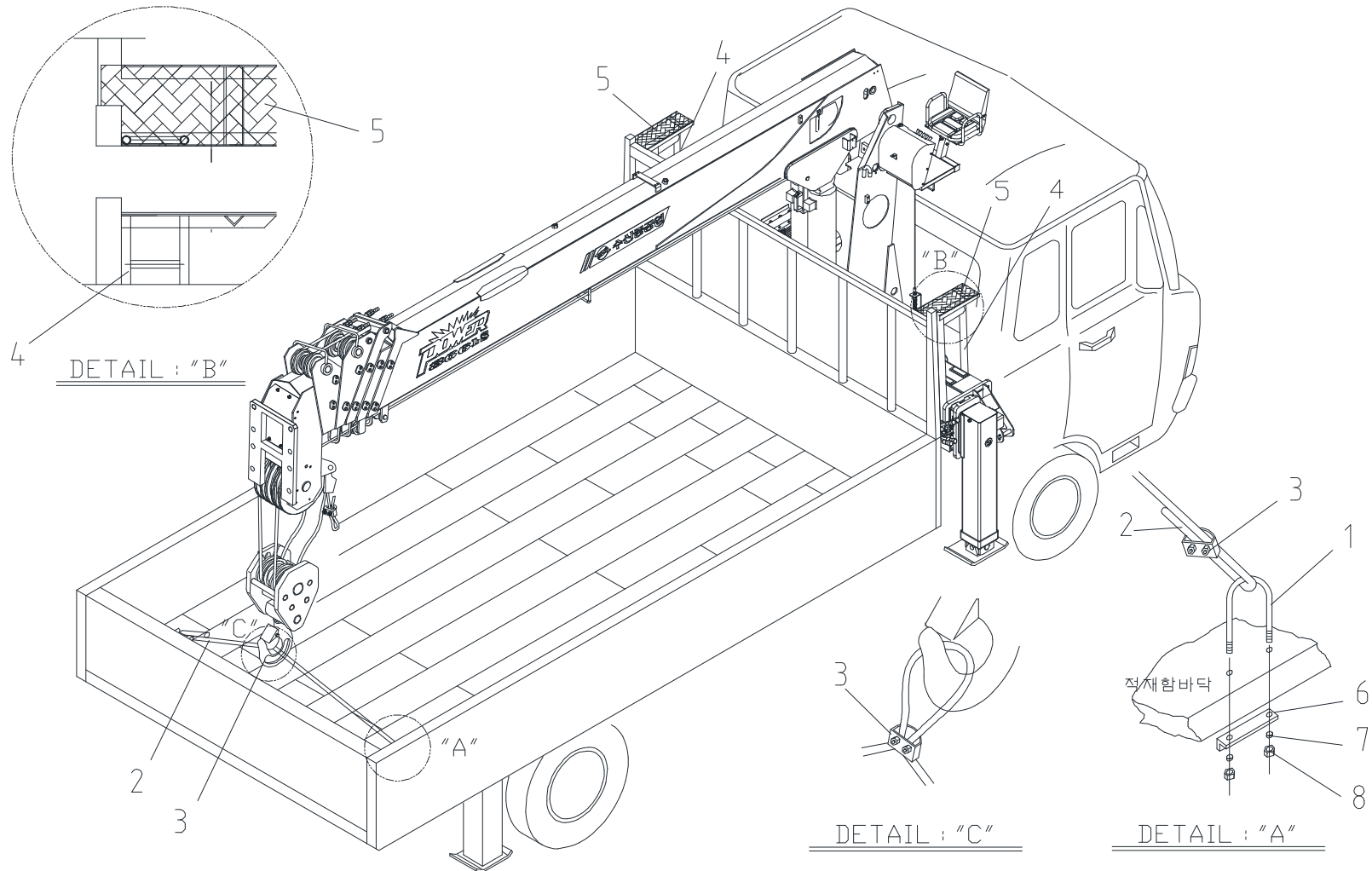
로딩 박스 파트 Fig. 9-5 SCS886 LOADING BOX PART
