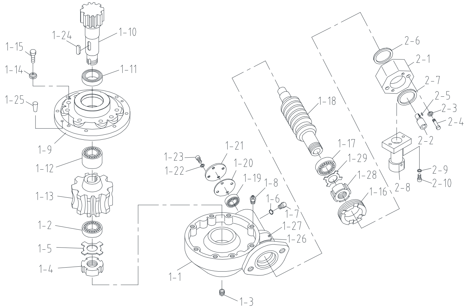
스윙 감속기 세트 Fig. 2-3 SCS886 SWING R/ G SET
