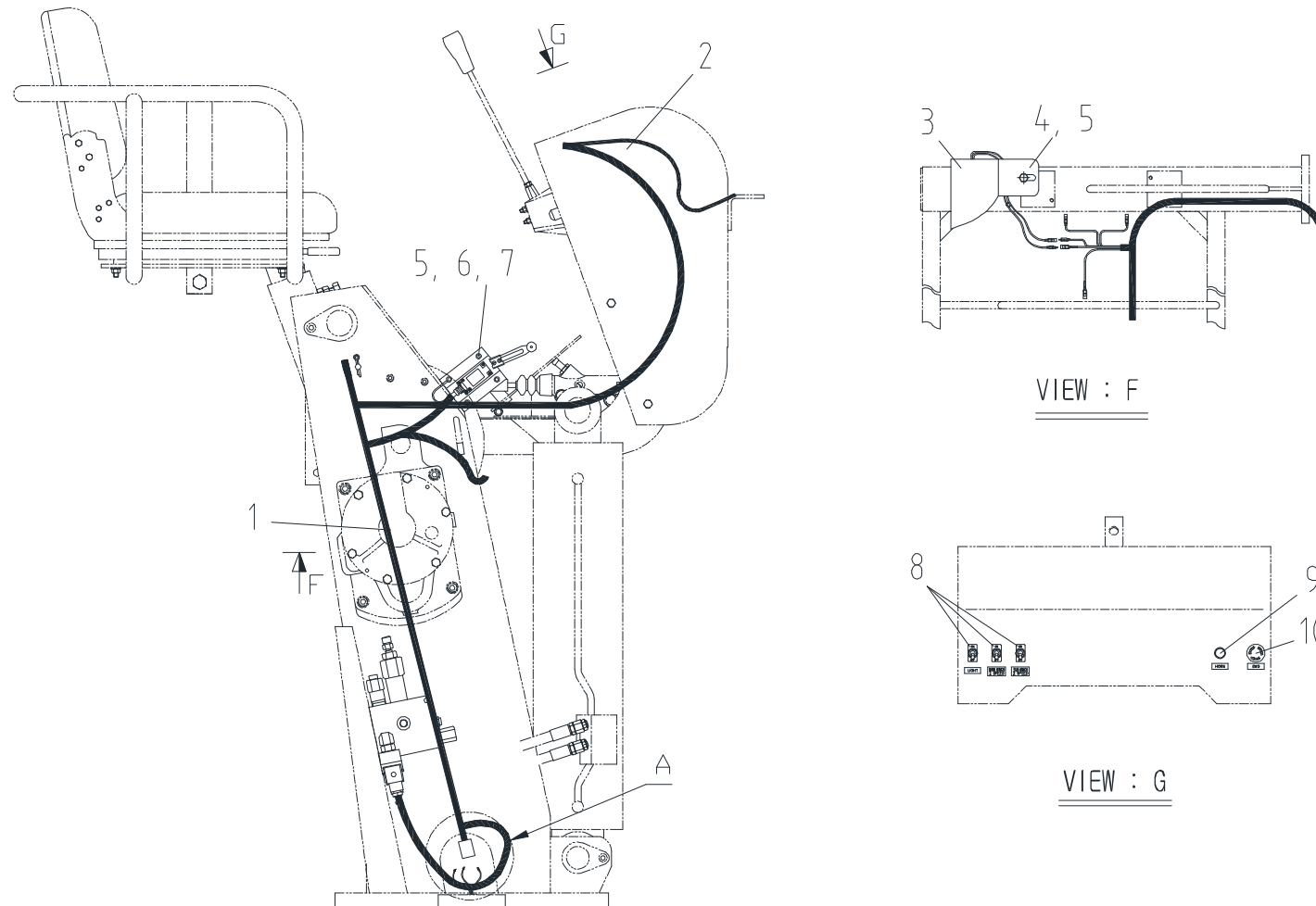
포스트 전선 Fig.10-2 SCS886 POST WIRING
