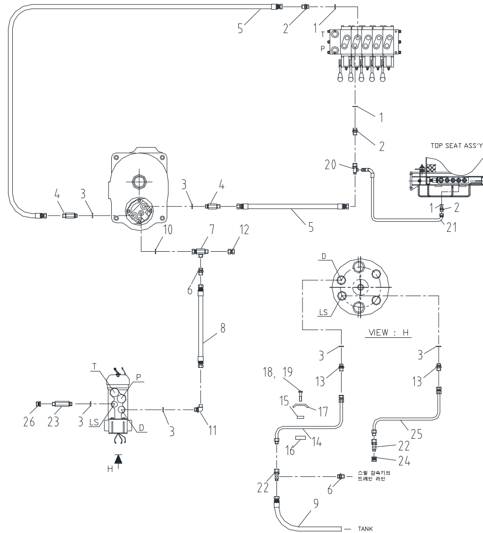
메인 윈치 배관 Fig. 5-3 SCS886 MAIN WINCH PIPING
